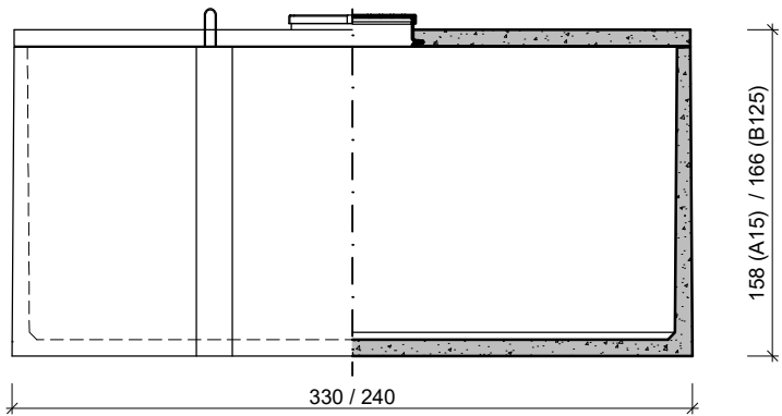
VUE FRONTALE / COUPE
